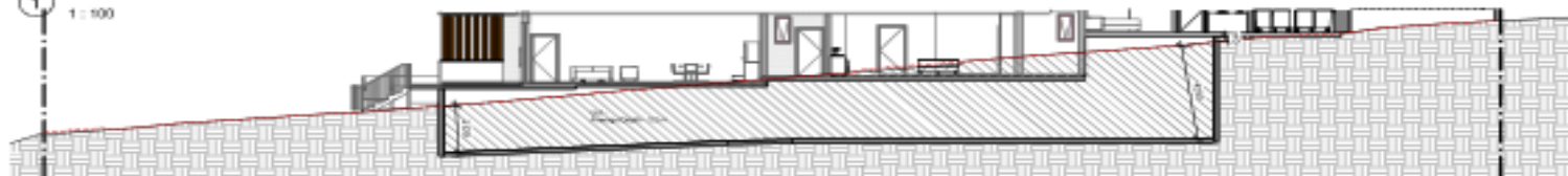
2 Cut & Fill - AA 1:100
